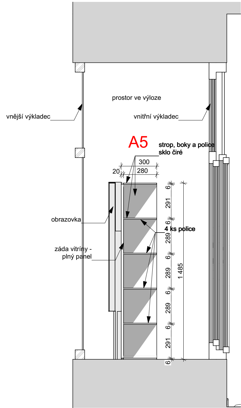
ŘEZ B-B'
