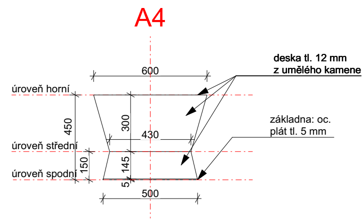
POHLED A-A'
