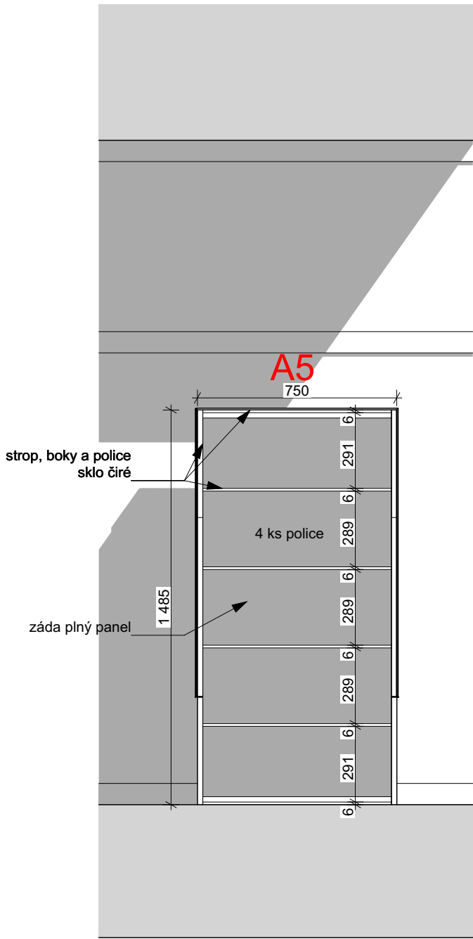
POHLED A-A'
