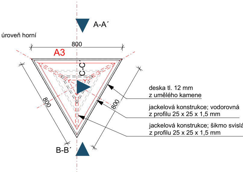
PŮDORYSY
