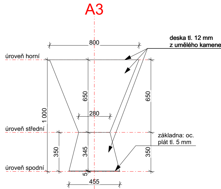
POHLED A-A'
