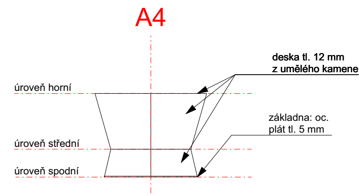
POHLED B-B'
