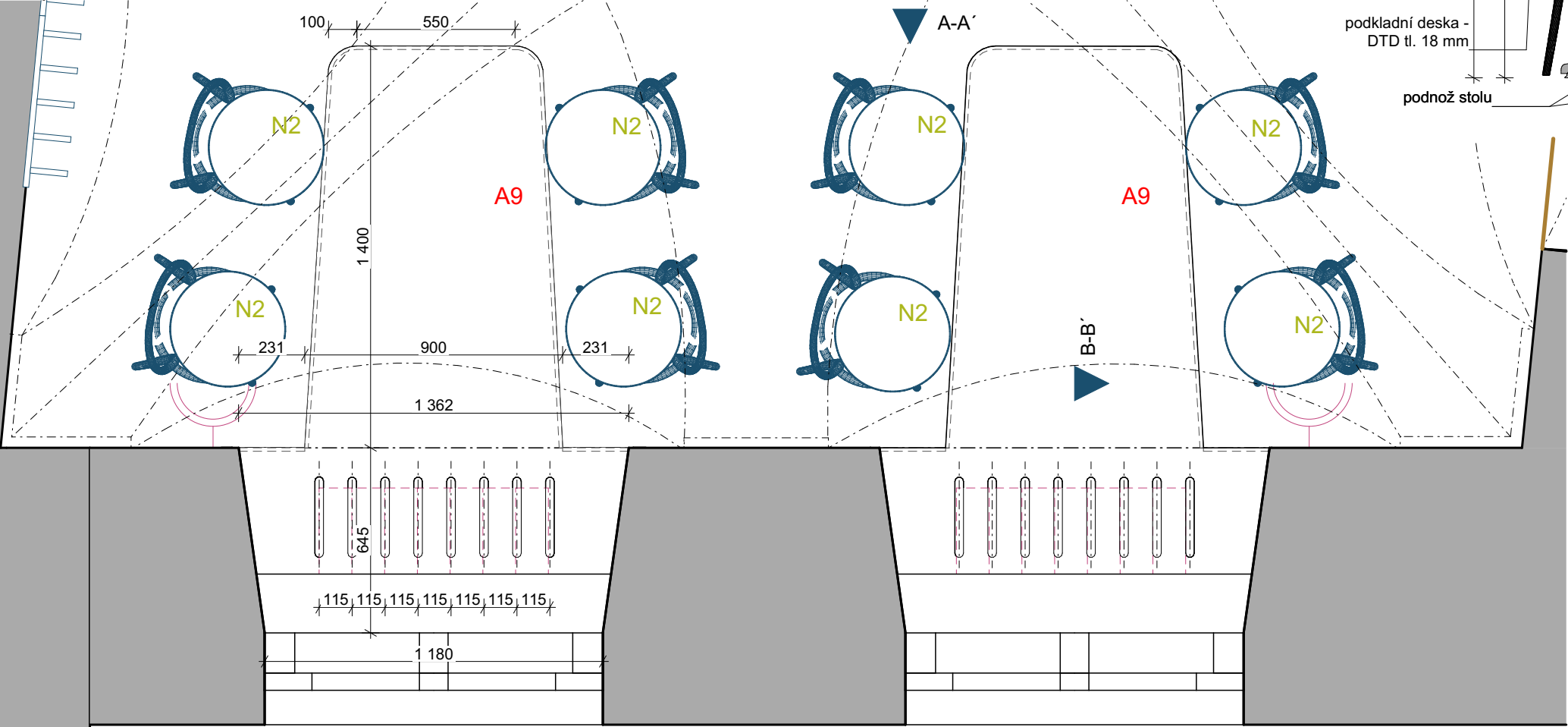
PŮDORYS
