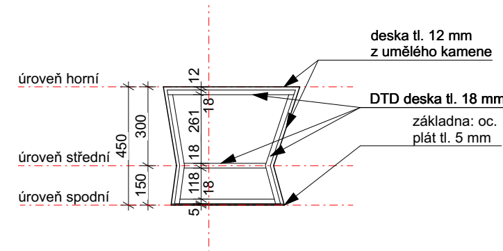
ŘEZ C-C'
